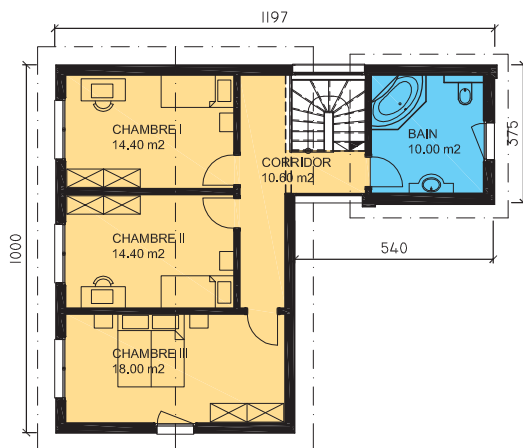
ETAGE
