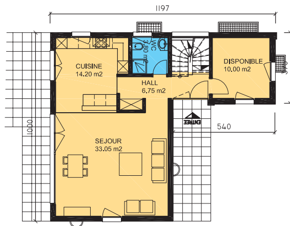
REZ-DE-CHAUSSEE
